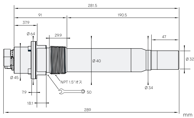
MGP241寸法
